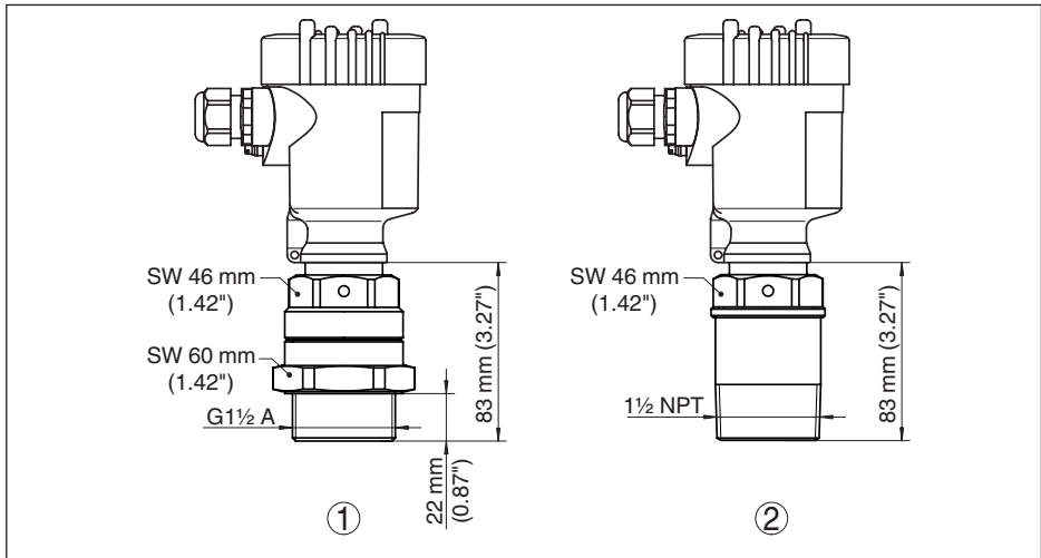
Abb. 45: VEGAMIP 61, innenliegende Hornantenne (Gewindeausführung)
