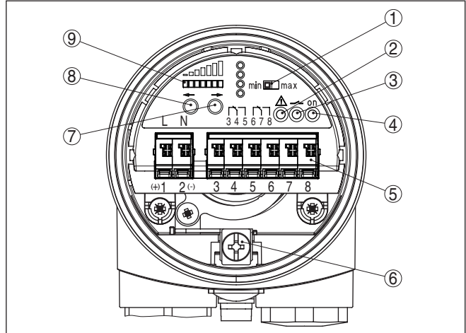
Abb. 23: Elektronikinsatz MP6X R (Empfängereinheit) - Relaisausgang
