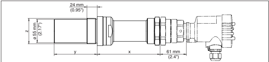
Abb. 50: Montageadapter mit Tubus (optional) für frontbündigen Einbau, für VEGAMIP 61 mit innenliegender Hornantenne, Gewindeausführung G1½ mit PTFE-Abdeckung (auch mit 1½ NPT-Gewinde)
