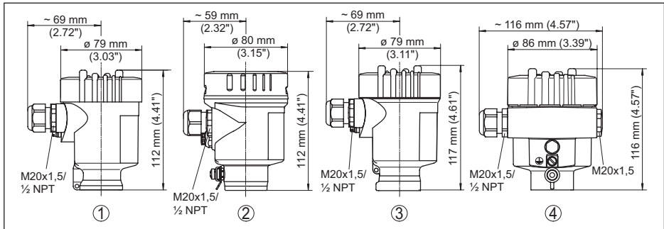
Abb. 44: Gehäuseausführungen
