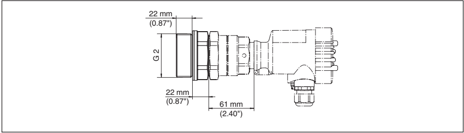
Abb. 48: Montageadapter mit Keramikabdeckung (optional) für VEGAMIP 61 mit innenliegender Hornantenne, Gewindeausführung G1½ mit PTFE-Abdeckung (auch mit 1½ NPT-Gewinde)
