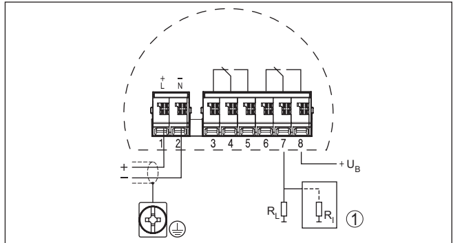
Abb. 22: Anschlussplan Empfängereinheit - VEGAMIP 61 (Receiver) bei Anschluss an eine SPS
