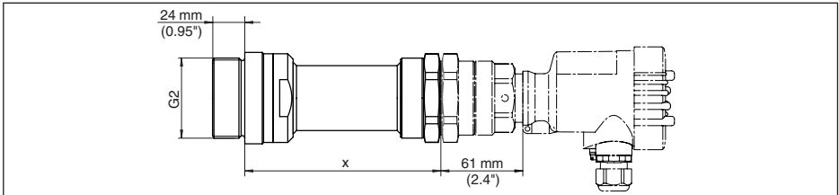
Abb. 49: Montageadapter mit Keramikabdeckung (optional) für VEGAMIP 61 mit innenliegender Hornantenne, Gewindeausführung G1½ mit PTFE-Abdeckung (auch mit 1½ NPT-Gewinde)
